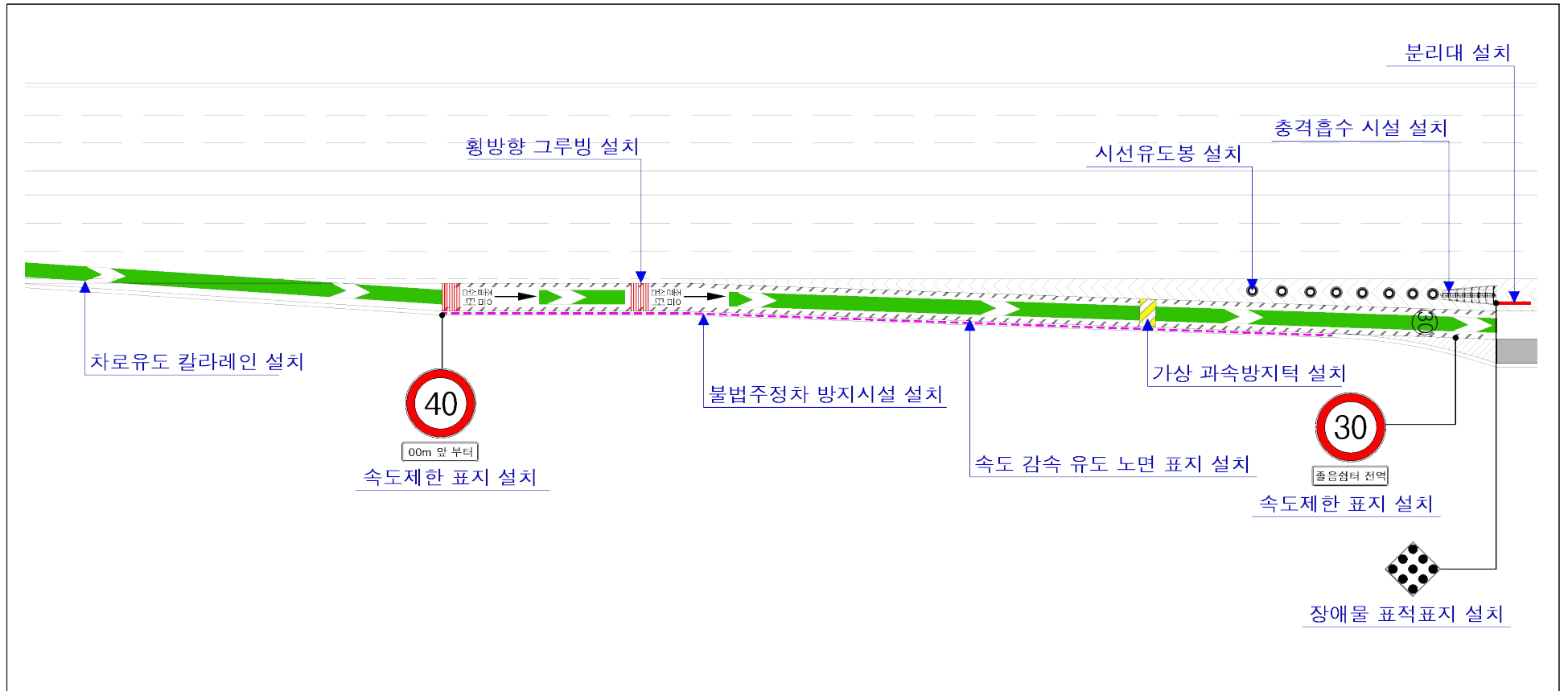
[별표 5]진입로 안전시설 종류 및 설치 위치
